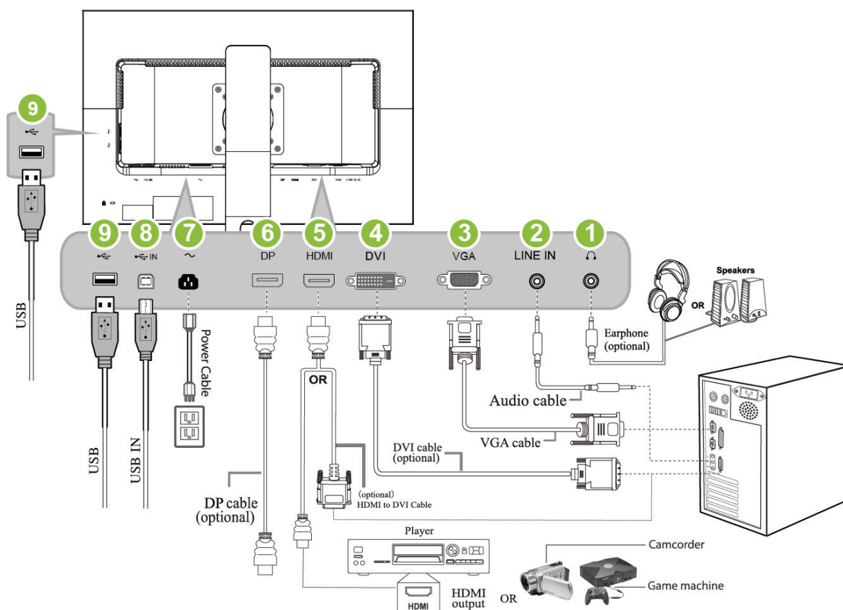
Figura 2. Branchement à un pc
